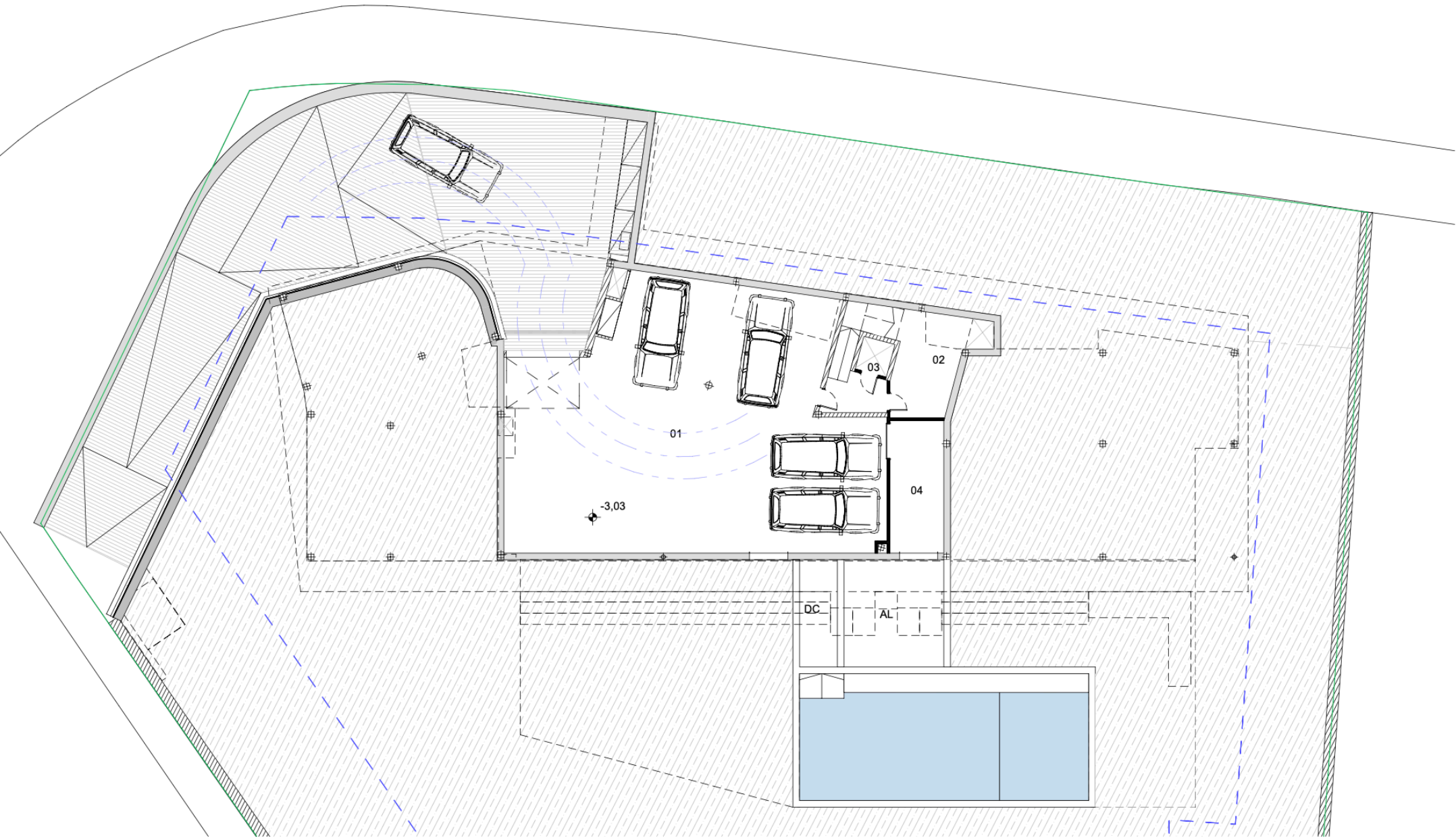
-1. Planta Sótano
