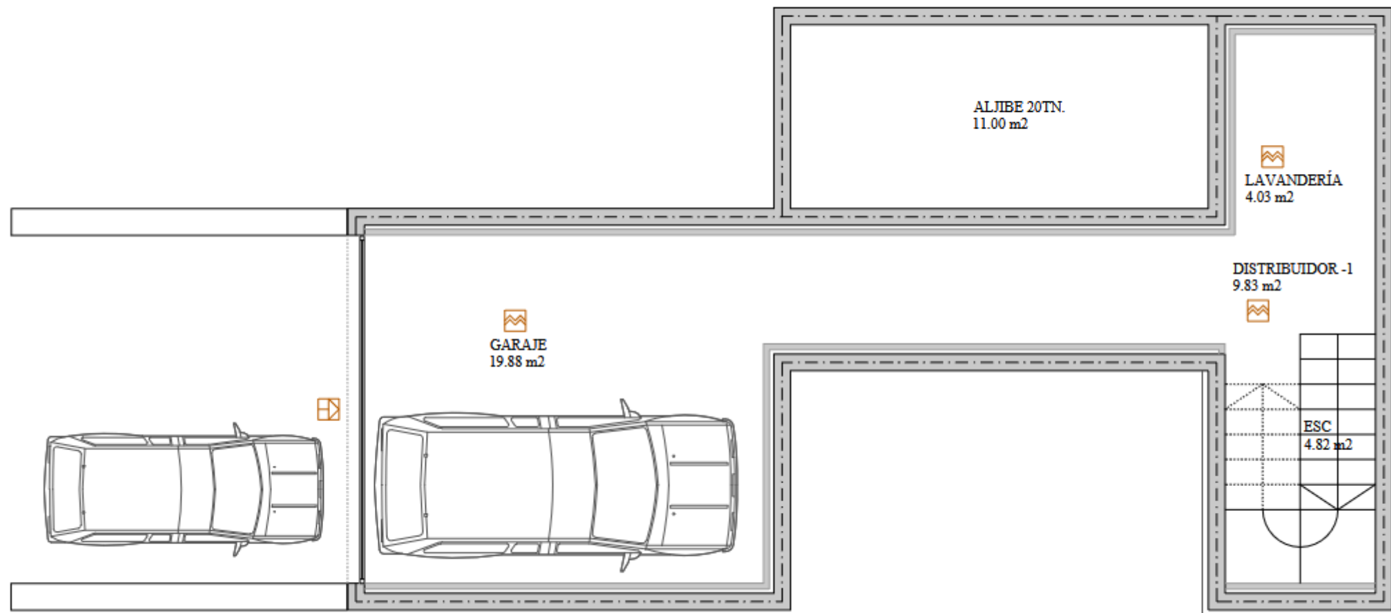
PLANTA SÓTANO. DH-HS2-HS3 SALUBRIDAD. 1/50
