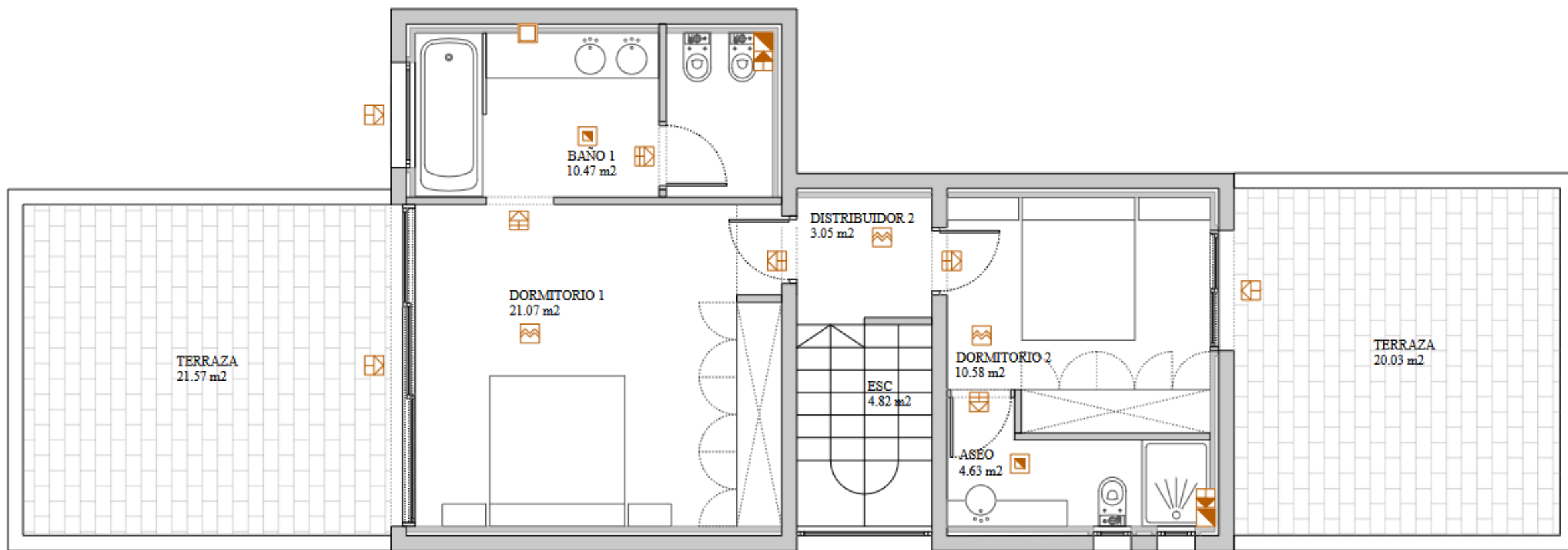
PLANTA PRIMERA. DH-HS2-HS3 SALUBRIDAD. 1/50
