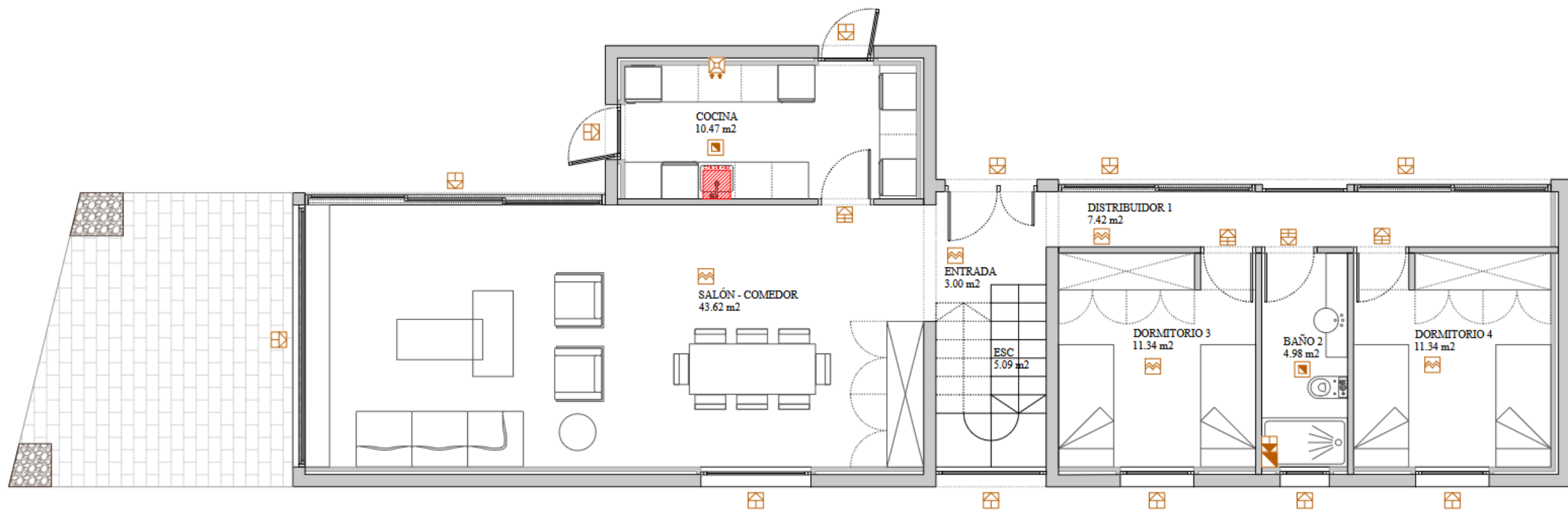
PLANTA BAJA. DH-HS2-HS3 SALUBRIDAD. 1/50
